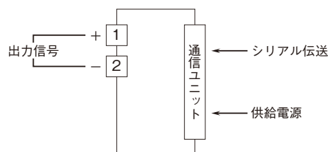
端子接続図
