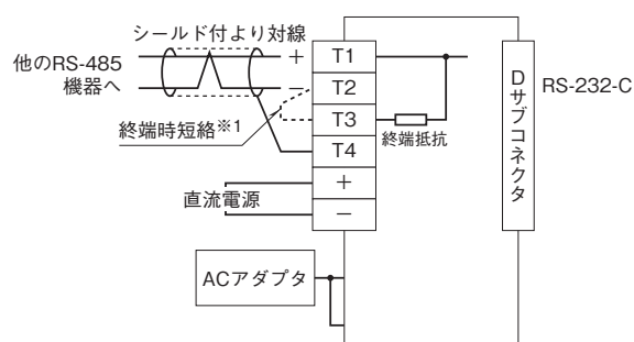
端子接続図
