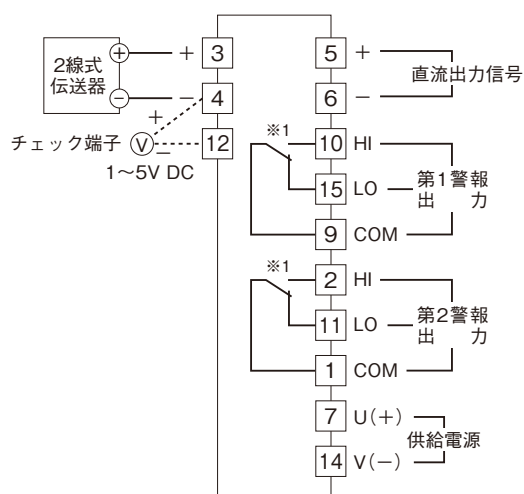
端子接続図
