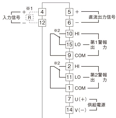
端子接続図
