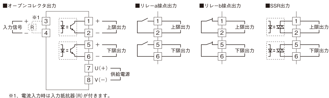
端子接続図
