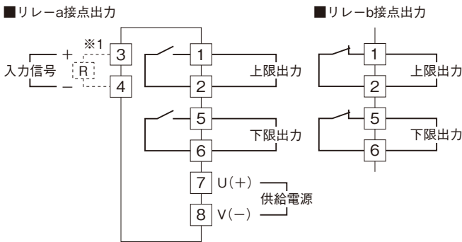
端子接続図
