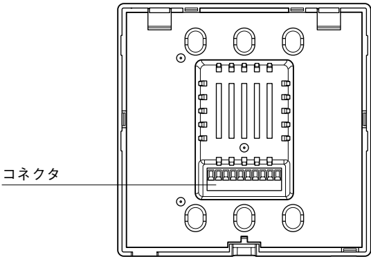
■背面図
