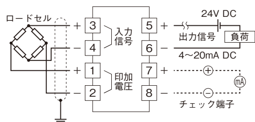
端子接続図
