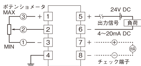
端子接続図
