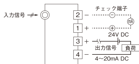
端子接続図
