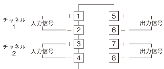
端子接続図
