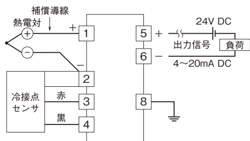
端子接続図
