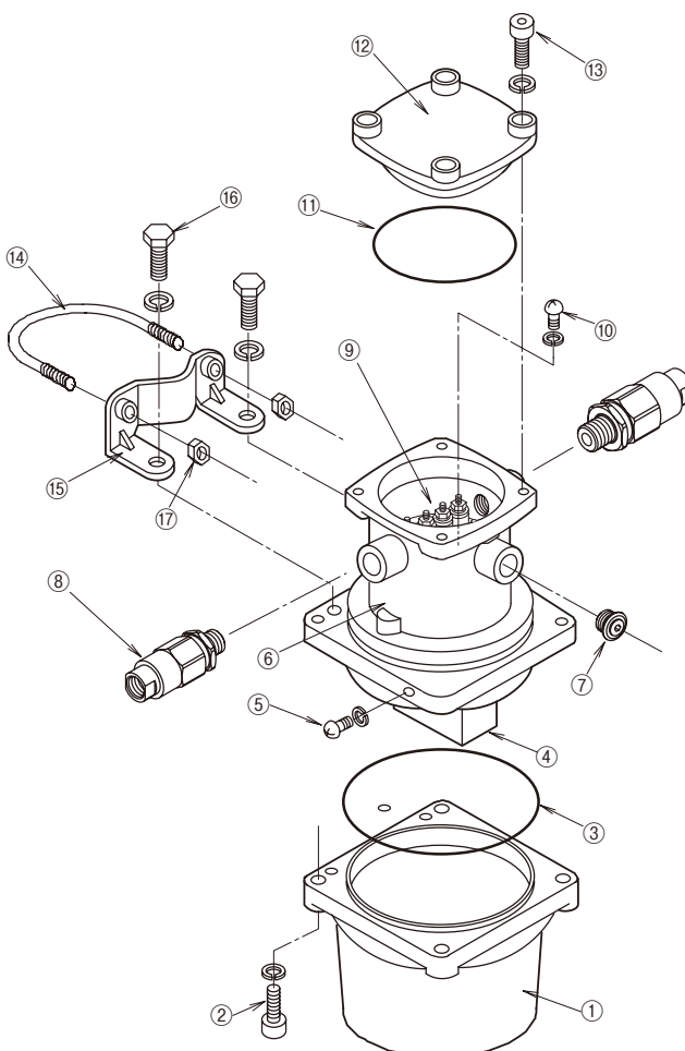
組立図 (収納タイプ A、B、E、F の場合)
