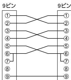
配線図
