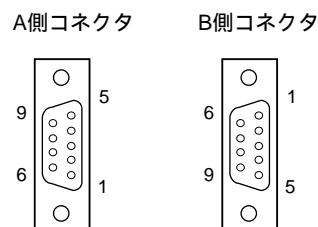
コネクタピン配列
