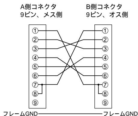
配線図
