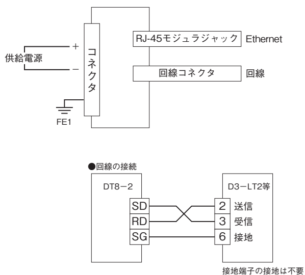
端子接続図
