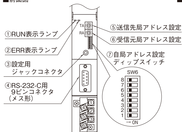
■前面図
