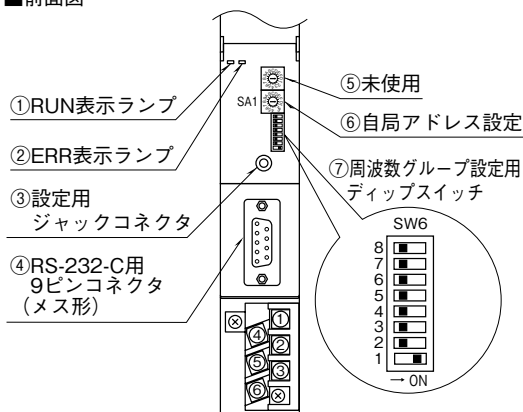
■前面図
