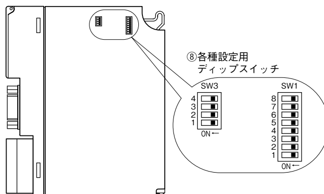
■側面図
