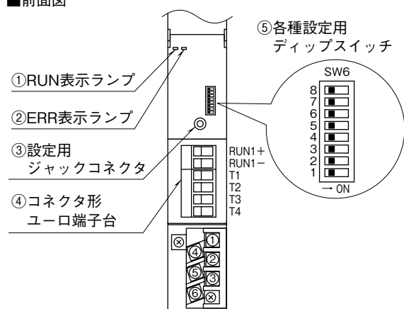
■前面図
