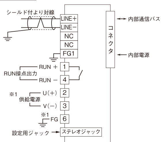
端子接続図
