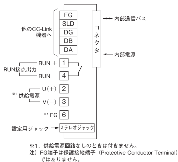
端子接続図
