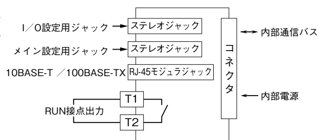
端子接続図
