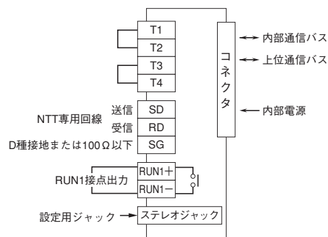
端子接続図
