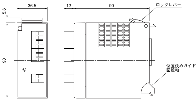
外形寸法図 (単位: mm)
