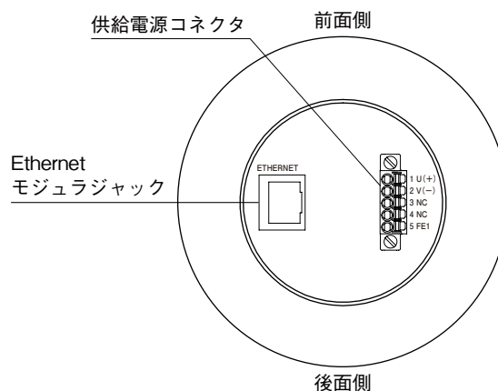
■底面図
