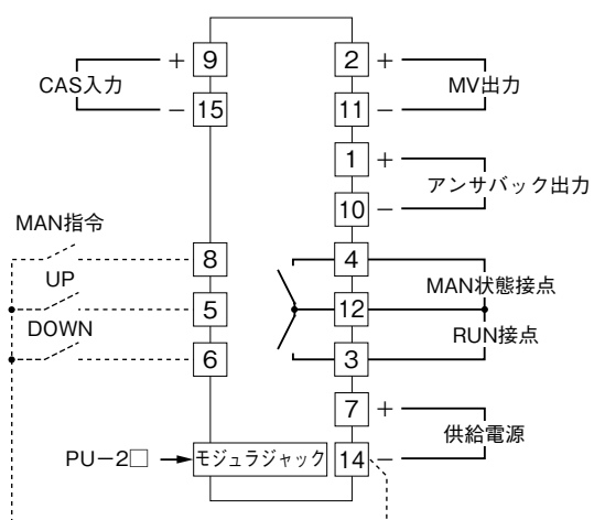
端子接続図
