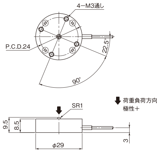
外形寸法図 (単位 : mm)
