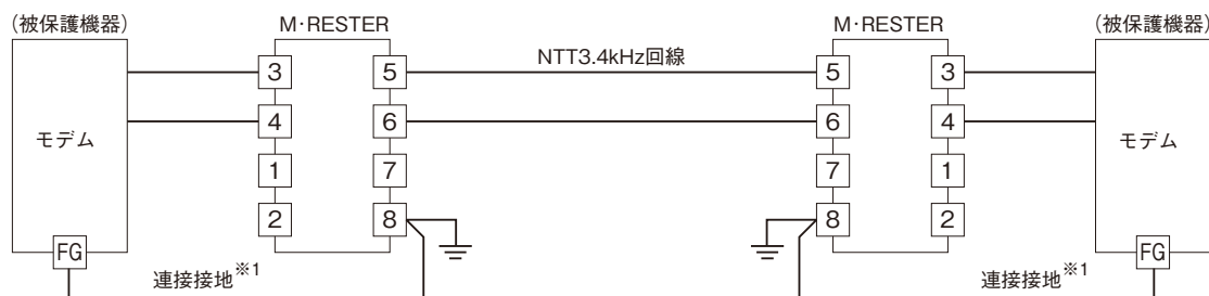
端子接続図
