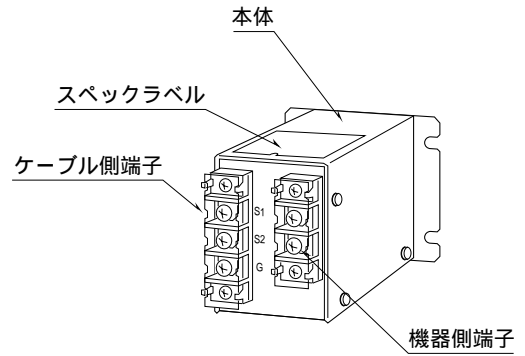
前面図
