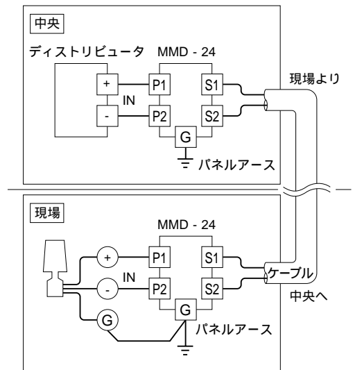
結線要領図
