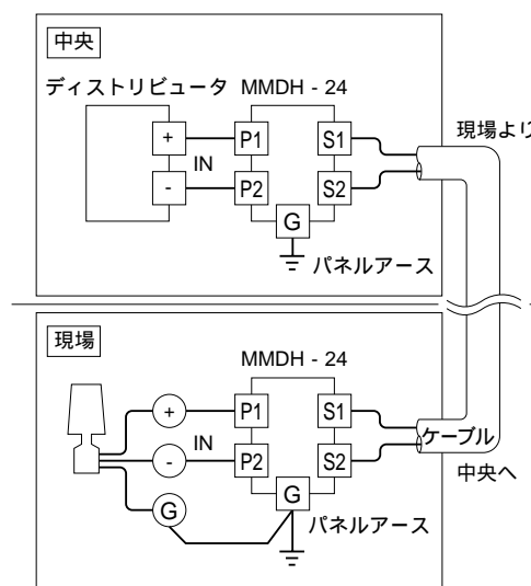
結線要領図
