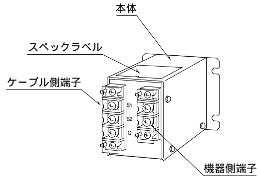
前面図
