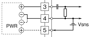
・交流カップリング時
