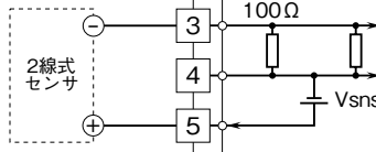
・外部DC電源使用時
