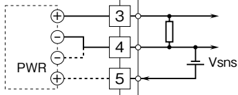
・交流カップリング時
