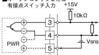
■オープンコレクタまたは有接点スイッチ入力
