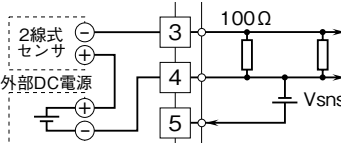
・外部DC電源使用時
