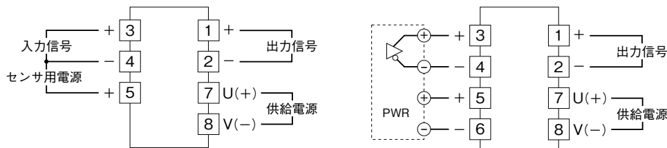
■RS-422ラインドライバ・パルス入力
