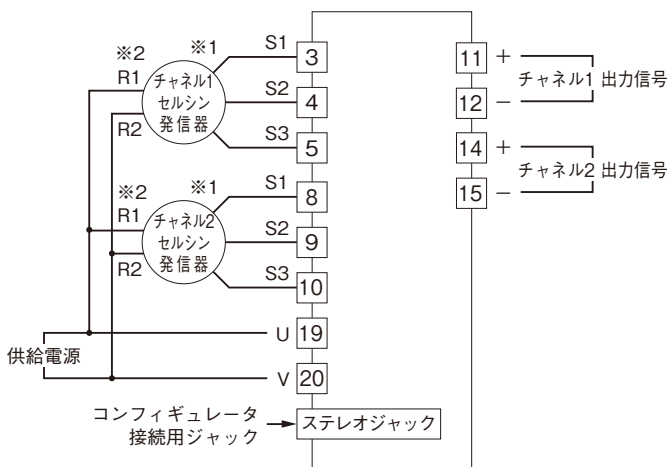
端子接続図
