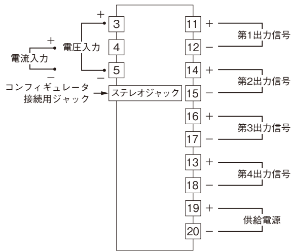
端子接続図
