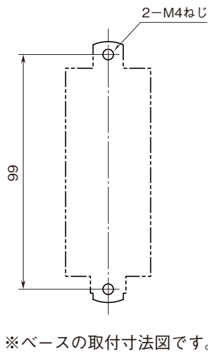
取付寸法図 (単位 : mm)
