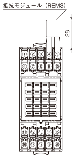
端子番号図 (単位 : mm)
