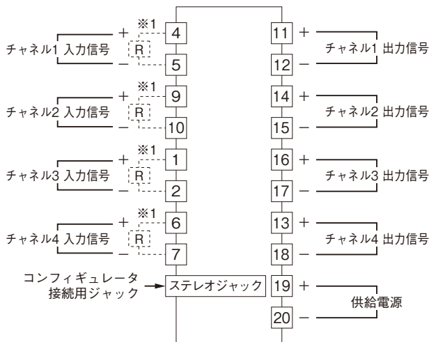
端子接続図
