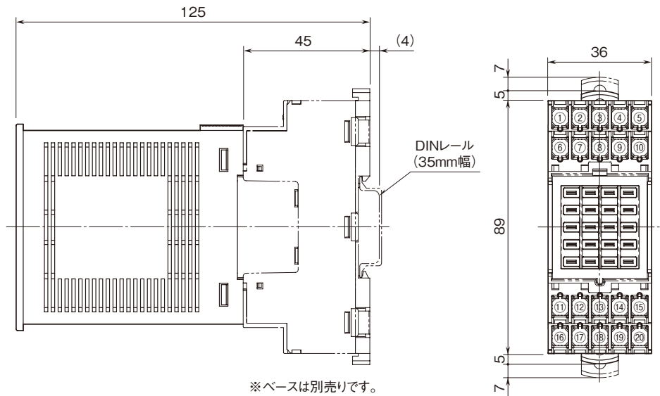
取付寸法図 (単位 : mm)
