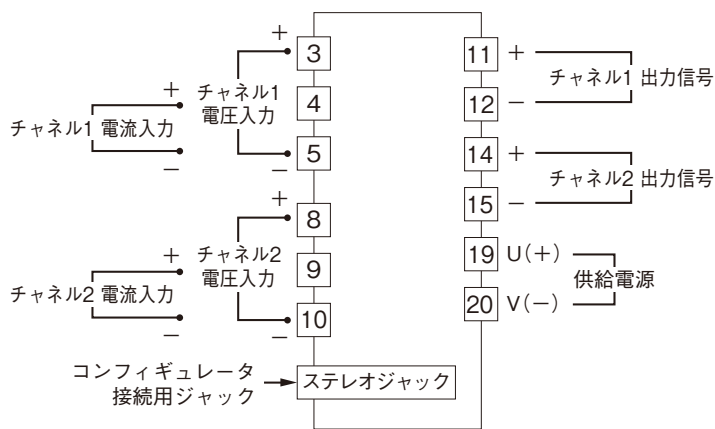
端子接続図
