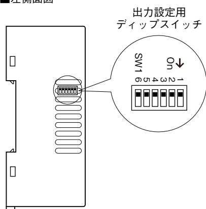
■左側面図
