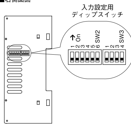
■右側面図
