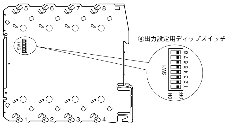
■側面図
