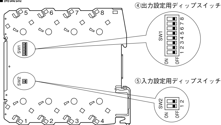
■側面図
