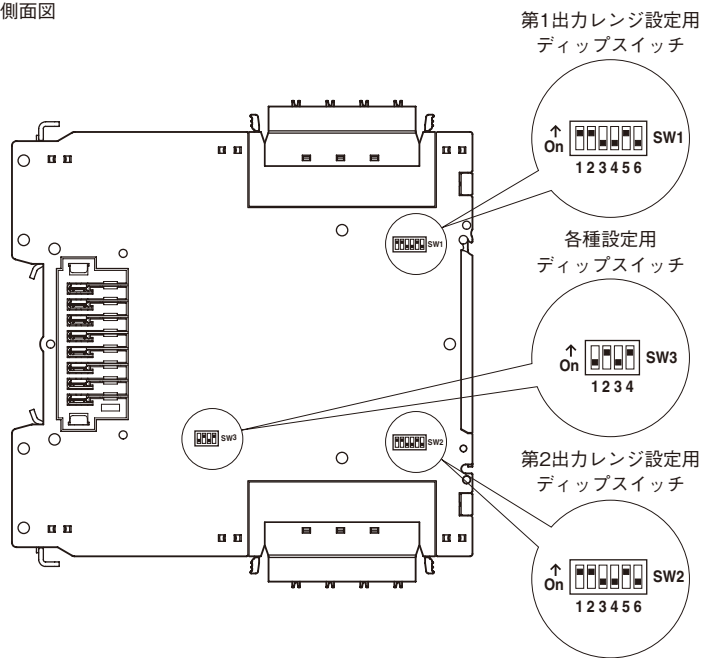
■左側面図
