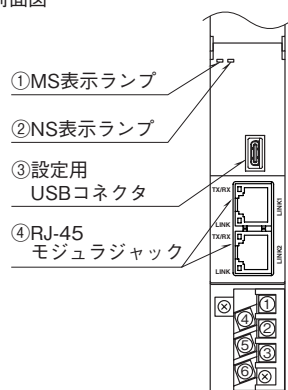
■前面図
