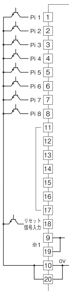
端子接続図
