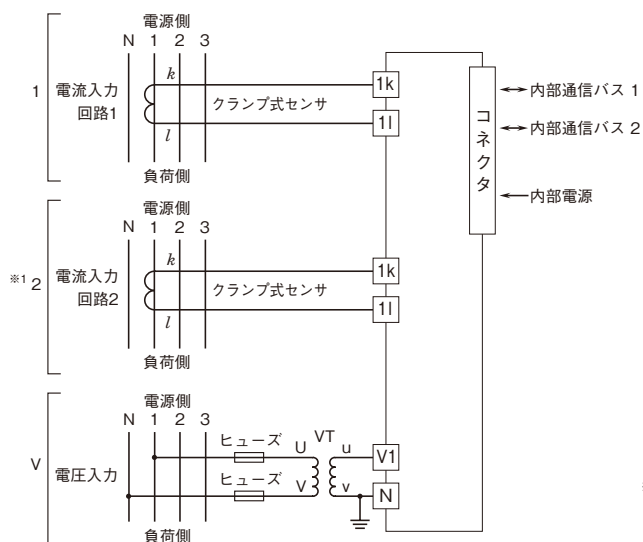
■三相4線 平衡負荷
