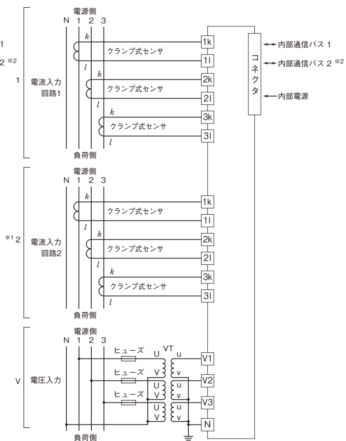
■三相4線 不平衡負荷3線
