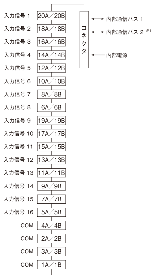
端子接続図
