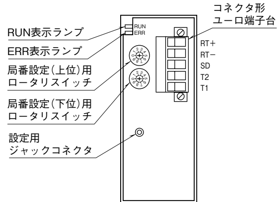
■前面図
