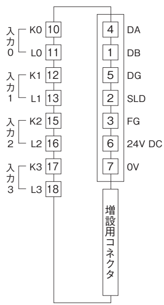
■入力部接続例
