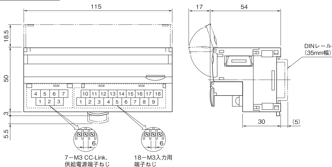
端子接続図
