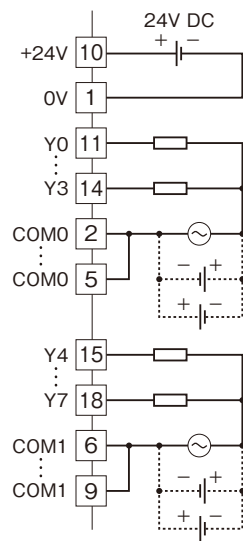
4点 1コモン
