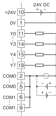
8点 1コモン
