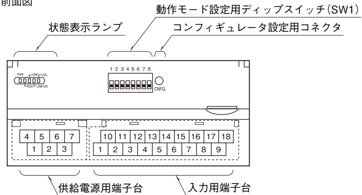
■前面図
