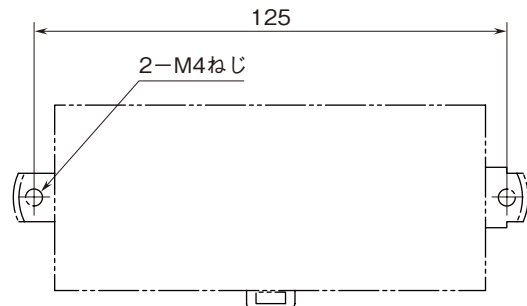
取付寸法図 (単位 : mm)
