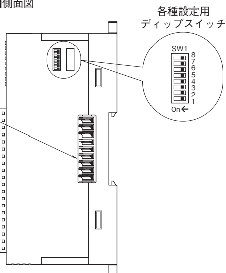
■側面図
