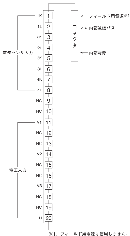
端子接続図
