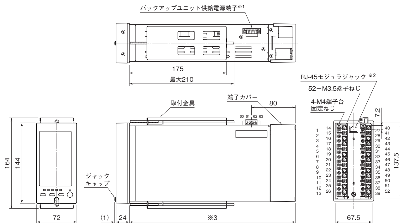
外形寸法図 (単位: mm)
